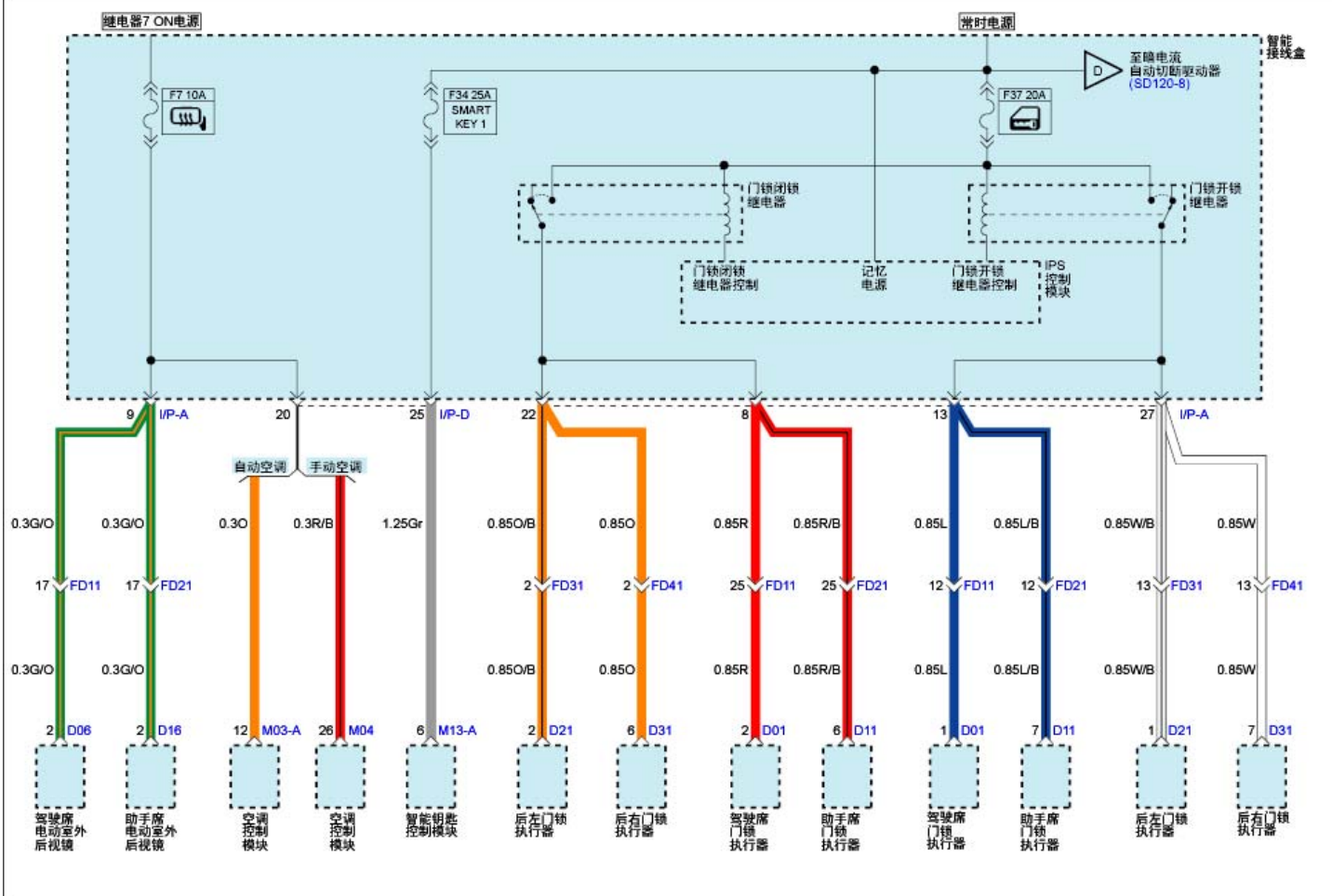
室内保险丝分布 (7)
